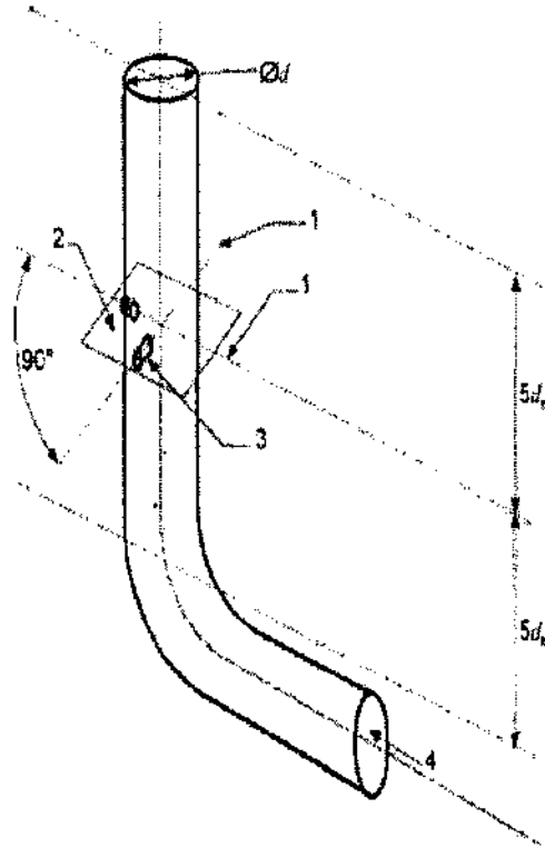
Şekil 1: Numune alma hattı ve düzlemi
