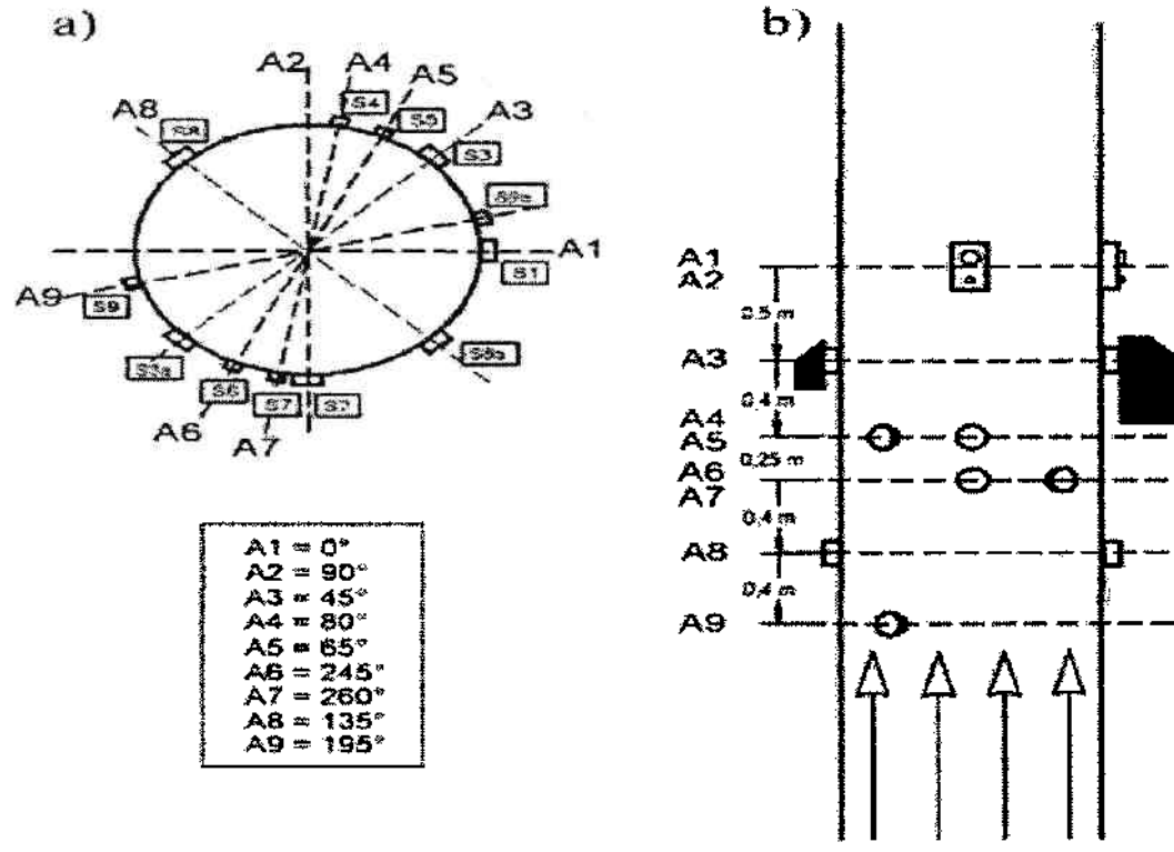
Şekil 3: Numune alma noktaları için örnek yerleşim planı
