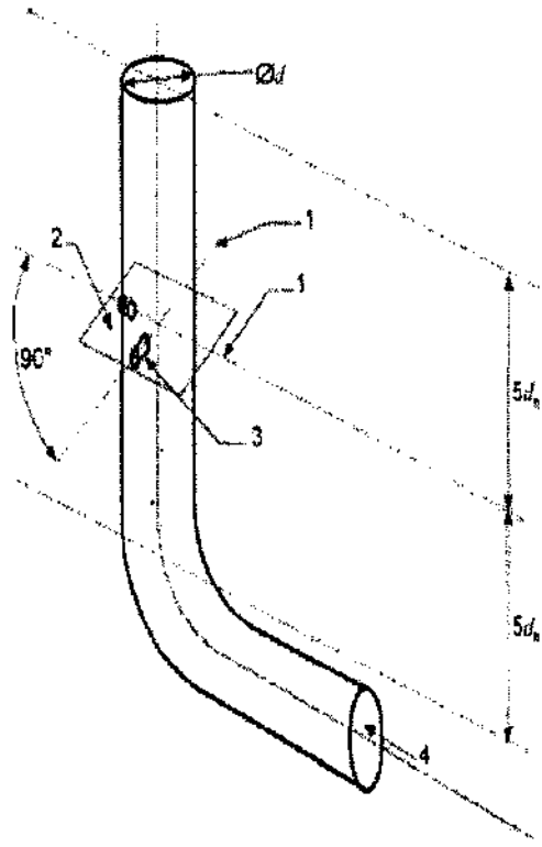
Şekil 1: Numune alma hattı ve düzlemi
